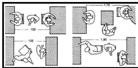
Gambar 6 Standar untuk Dimensi Ruang Gerak (Sumber: Ernst dan Peter Neufert, 2002: 3)
