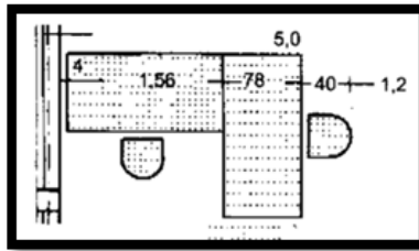
Gambar 3 Standar untuk Dimensi Ruang Pengelola (sumber: Ernst dan Peter Neufert, 2002: 13)
