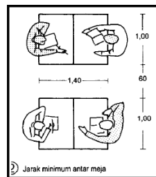
Gambar 5 Standar untuk Dimensi Ruang Baca (Sumber: Ernst dan Peter Neufert, 2002: 3)
