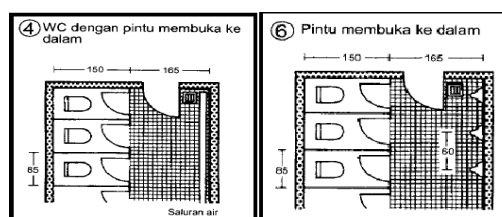
Gambar 2 Standar Dimensi Toilet
