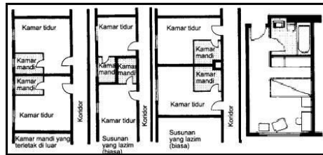
Gambar 8 Standar Untuk Denah Kamar Penginapan (sumber: Ernst dan Peter Neufert , 2002: 128)
