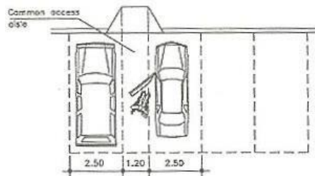
Gambar 12 Standar Dimensi mobil
