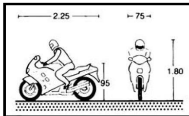
Gambar 11 Standar Dimensi Sepeda Motor
